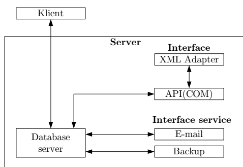
Figur 32: Arkitektur i Sap Business One, frit efter [SAP05a]
